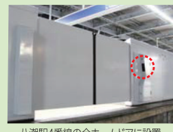
八潮駅4番線の全ホームドアに設置されたレーザー光線方式3Dセンサー ※○がセンサー部分
