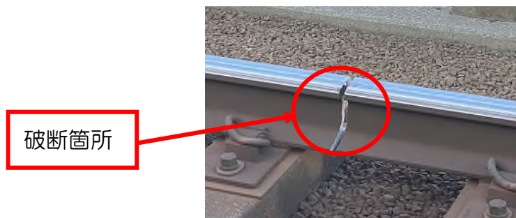
破断したレール側面の様子
