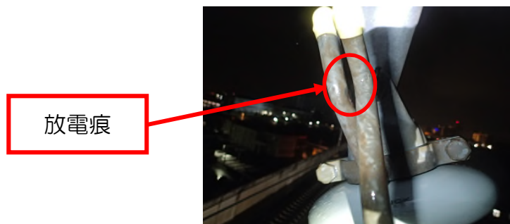
放電痕が残る電車線設備
